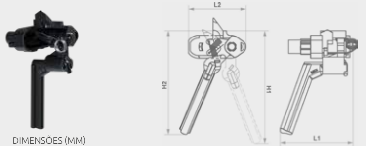
DIMENSÕES (MM)
