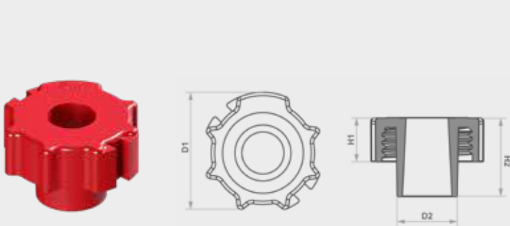
DIMENSÕES (MM)
