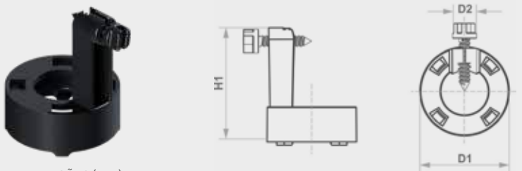
DIMENSÕES (MM)
