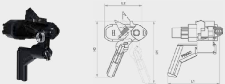
DIMENSÕES (MM)
