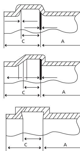
Diseño de ranuras típicas de campanas con juntas de anillo de sello elastomérico.
