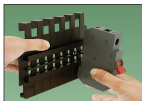
Disjuntor DIN
