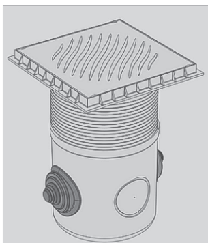
Exemplo da Caixa de Passagem Elétrica com prolongador
